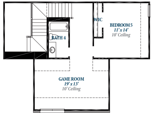
OPTIONAL BEDROOM 5
