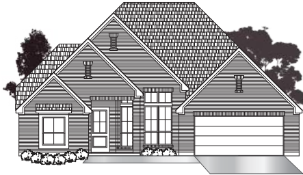
• ELEVATION A1 •
